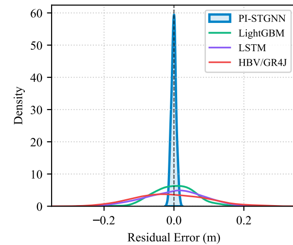
(b) Residual Error ( y - \hat{y} )
