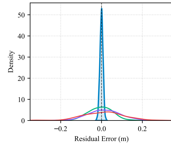
(f) Residual Error ( y - \hat{y} )
