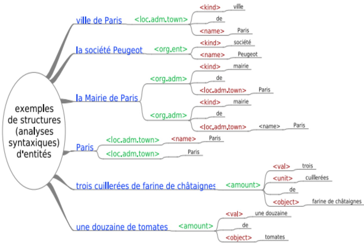
FIG. 1.3: Exemples d'entités.
