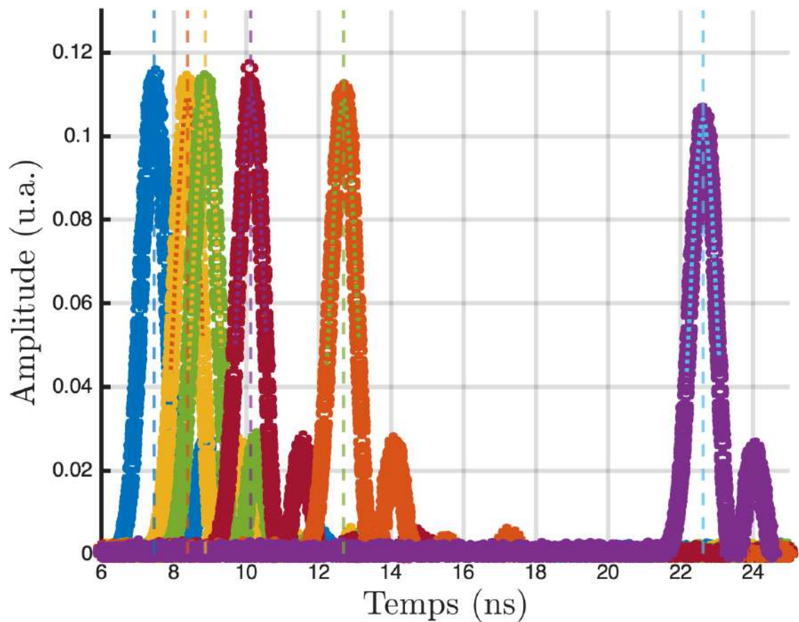
FIGURE 8 – Données de la dérivée des impulsions de chaque longueur de câble BNC RG-58, avec les ajustements paramétriques de type poly4 représentés par les lignes pointillées. La position temporelle du pic de la dérivée de l'impulsion est utilisée pour déterminer le temps d'arrivée du signal.
