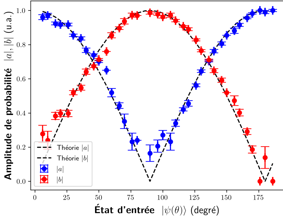
FIGURE 20 – R  sultats de l'amplitude de probabilit   pour le trajet de polarisation |H\rangle \rightarrow |R\rangle \rightarrow |V\rangle \rightarrow |L\rangle . Les donn  es sont calcul  es    partir de la partie r  elle de la valeur faible par les   quations 123 et 124. Les courbes th  oriques provenant des amplitudes de probabilit  s de l'  quation 150.
