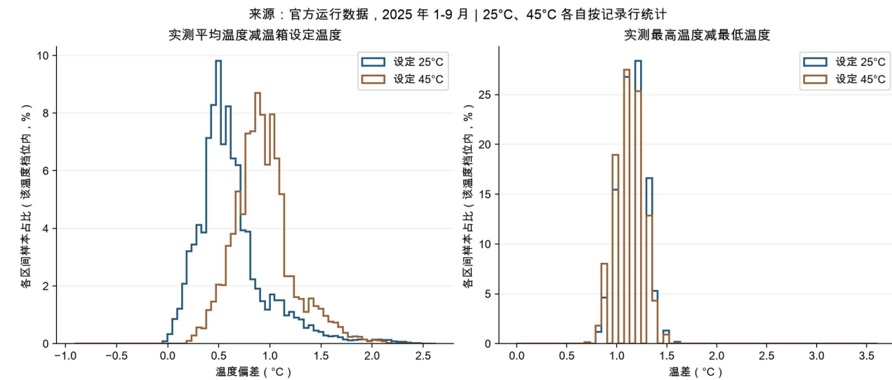
图 2 平均温度偏差与最高减最低温差的分布。来源为全部官方运行记录，25℃、45℃ 分别计算档位内部样本百分比，未按日历时间补齐缺失记录。
