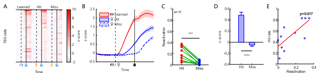
图 3.9 迁移学习的细胞重激活
