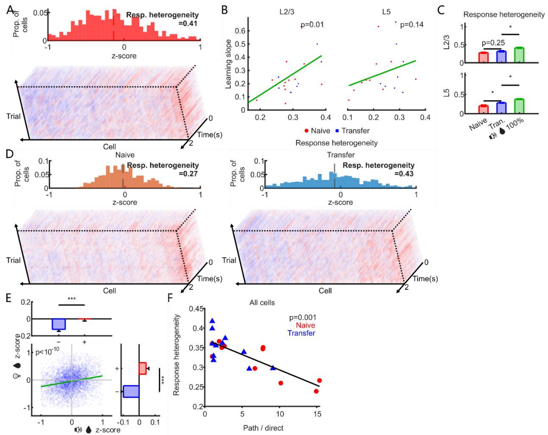
图 3.16 迁移与初始的响应异质性
