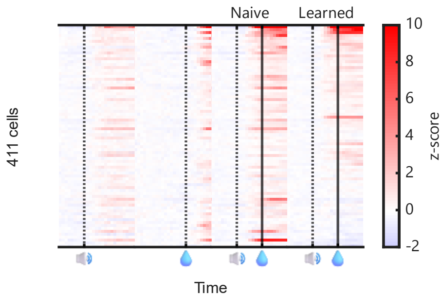
图 3.6 声水初始学习前后基本轮廓
