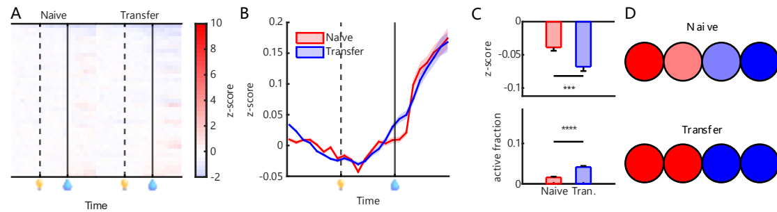
图 3.10 迁移与初始光水的总体活跃度
