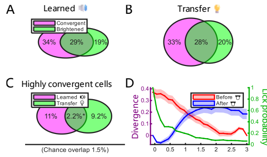
图 3.25 静息态自发舔水前后
