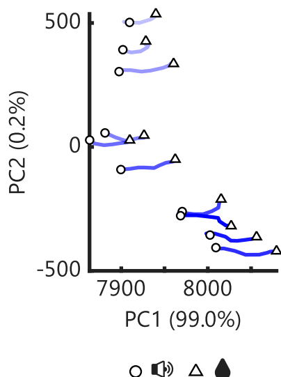
图 3.8 状态切换对全局状态空间的影响
