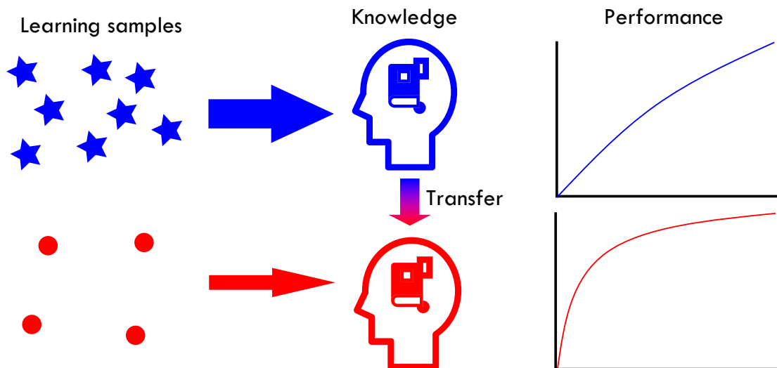
图 1.1 迁移学习
