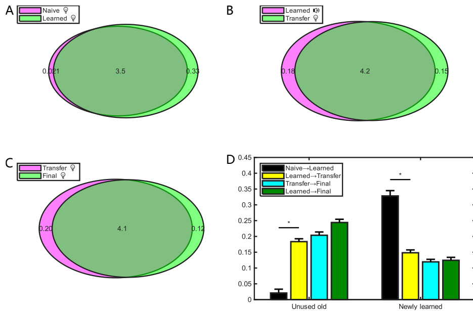
图 3.22 迁移学习的共享与新增知识量
