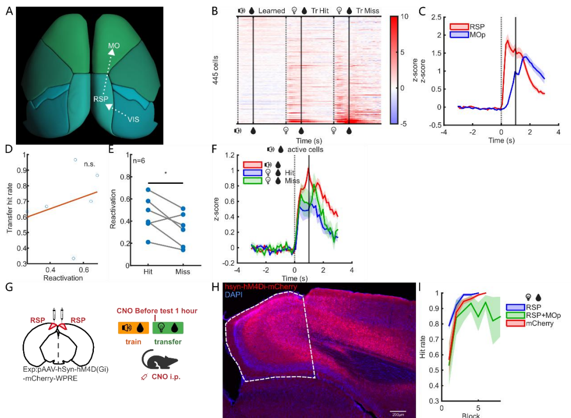
图 3.19 RSP 位于 VIS 与 MO 之间并偏向视觉相关上游输入
