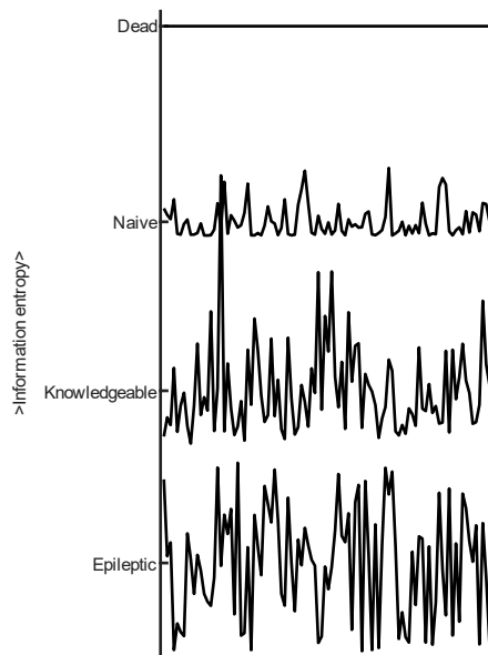
图 3.20 信息量计算
