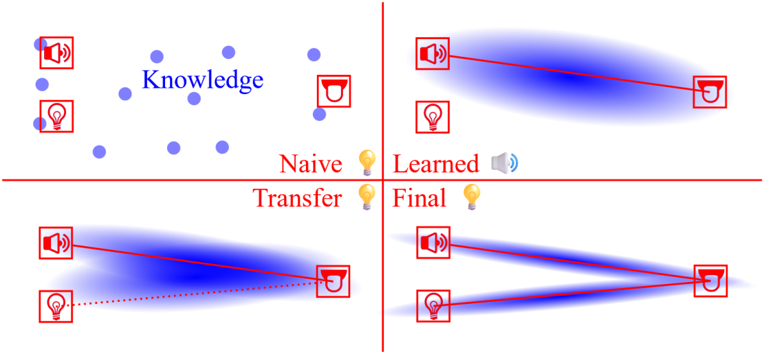
图 3.23 迁移学习的知识分布模型
