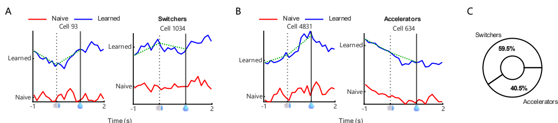
图 3.7 状态切换的两种可能性
