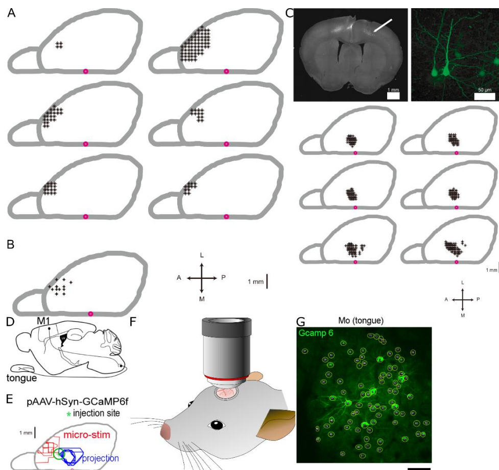
图 3.5 初级运动皮层钙成像
