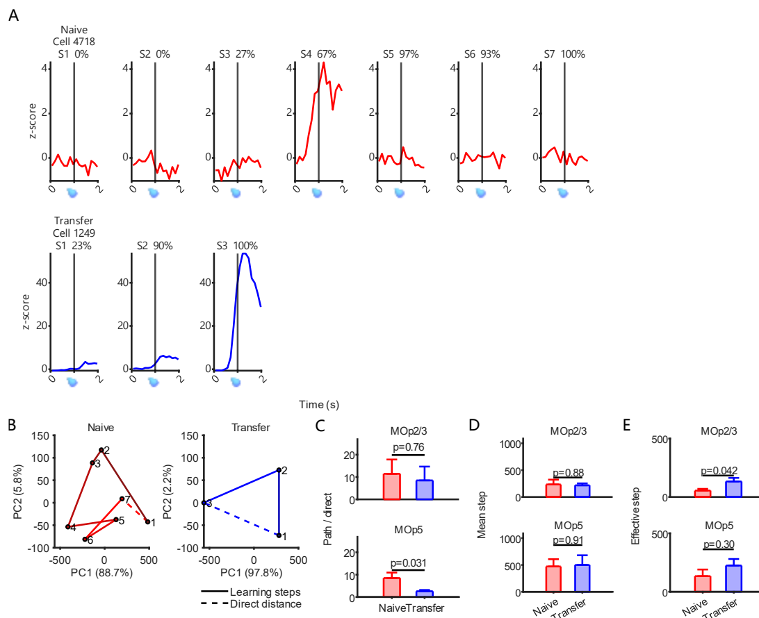
图 3.15 迁移学习走直线，不绕路
