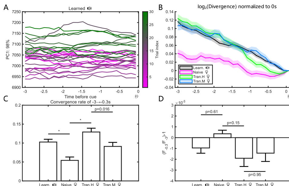
图 3.24 提示前的静息态自发收敛
