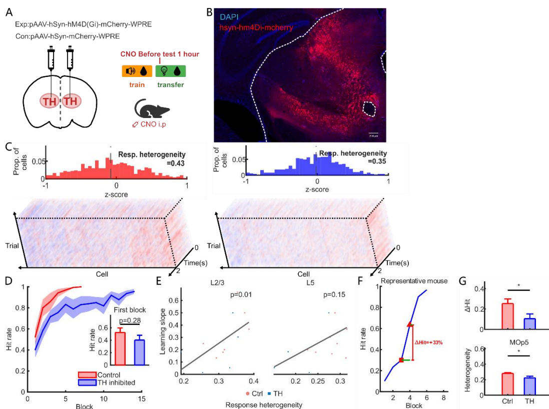
图 3.17 TH 抑制影响学习速度和响应异质性
