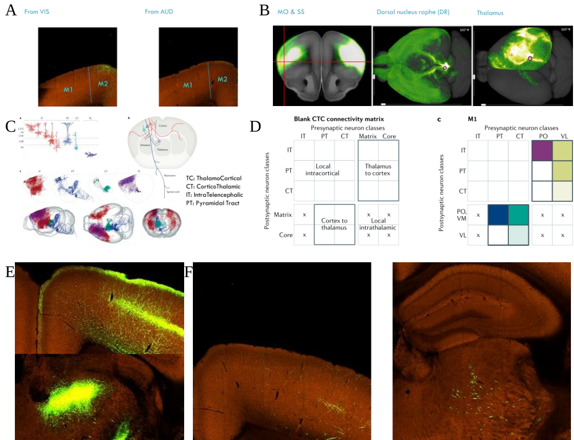
图 1.4 MOp 的上游投射关系
