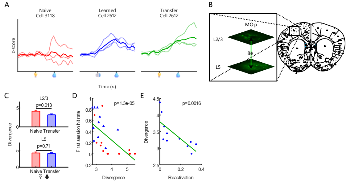
图 3.11 迁移的回合间稳定性
