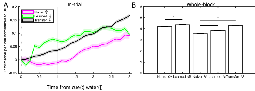
图 3.21 学会后信息量增加
