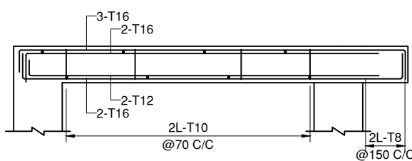
B7:230x450
