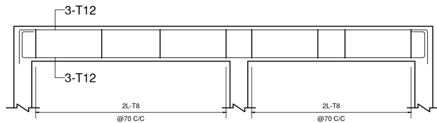
B1:230x450
