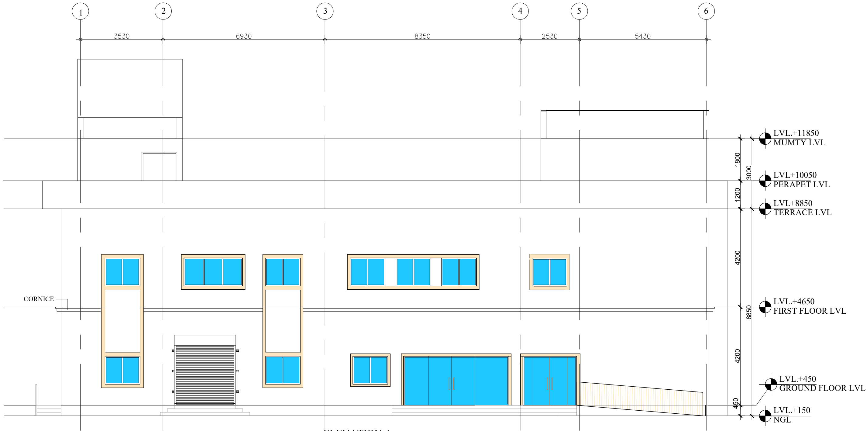
ELEVATION A
