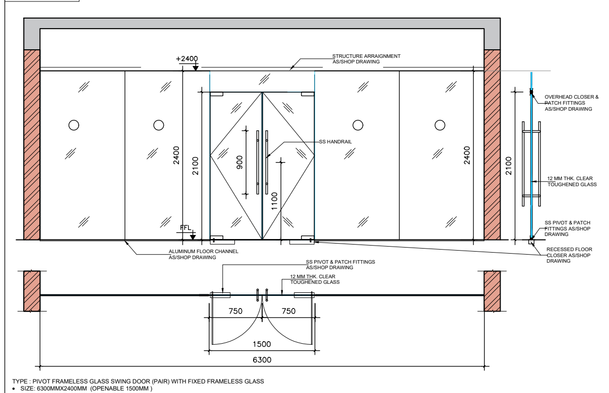
DOOR-GDW
