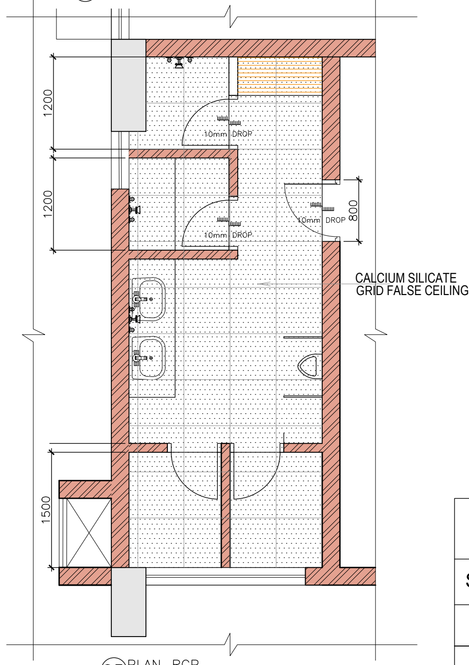
03 PLAN_RCP
