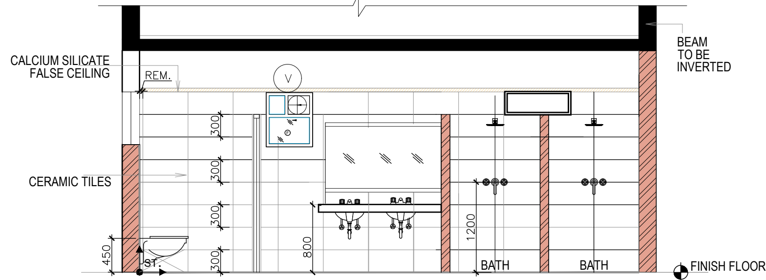
E3 ELEVATION
