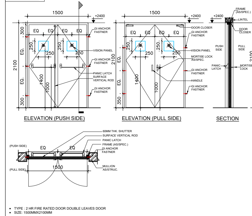
DOOR-FD
