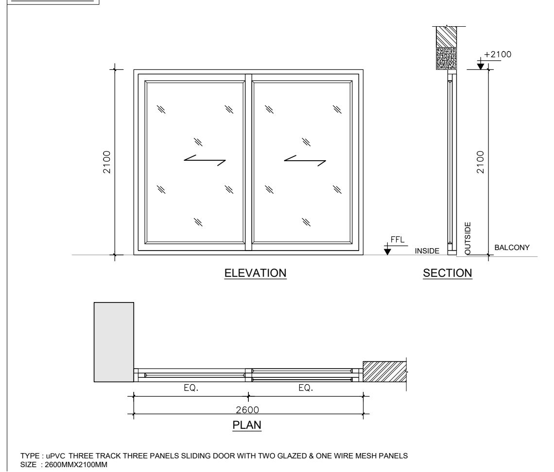
DOOR-DW1
