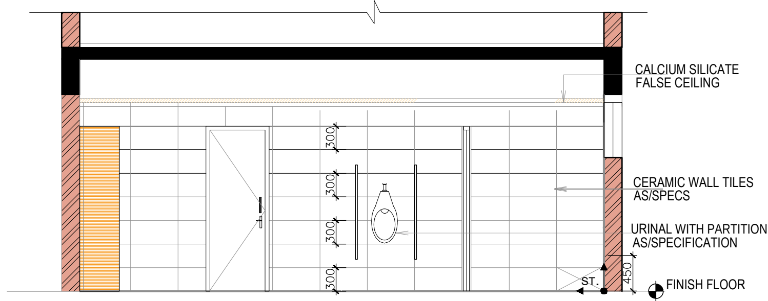
E2 ELEVATION
