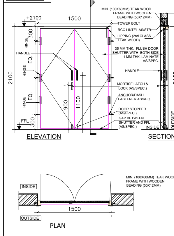
DOOR-D4
