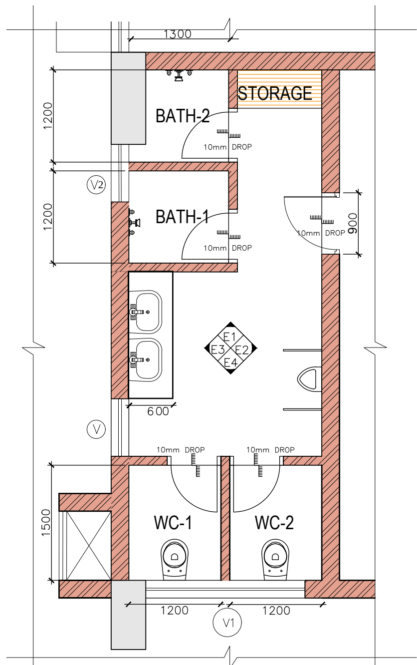
01 PLAN
