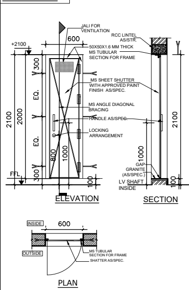
DOOR-SD2
