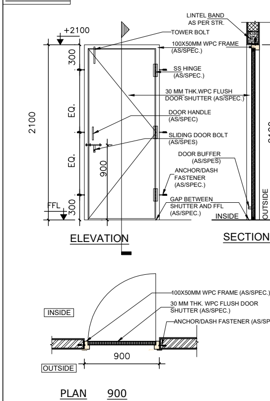
DOOR-D1
