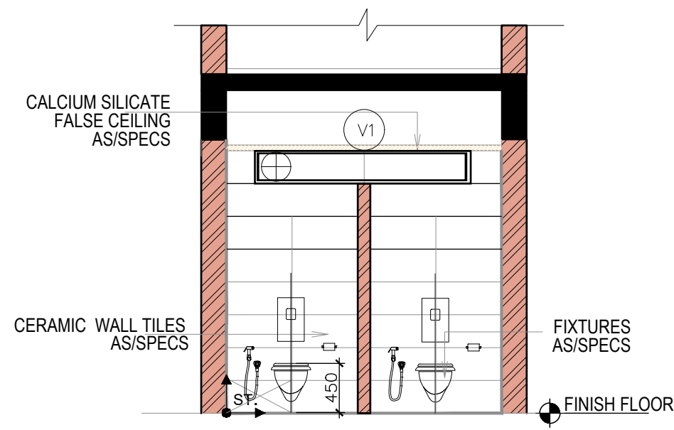
E4 ELEVATION
