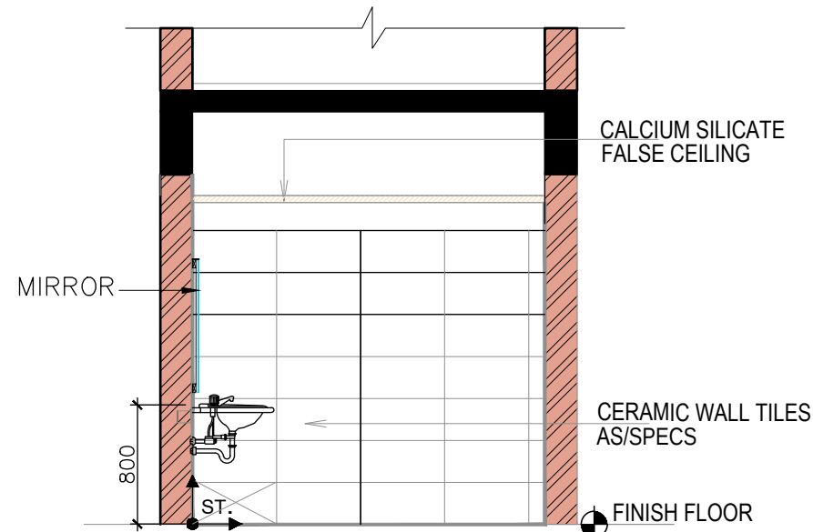
E1 ELEVATION
