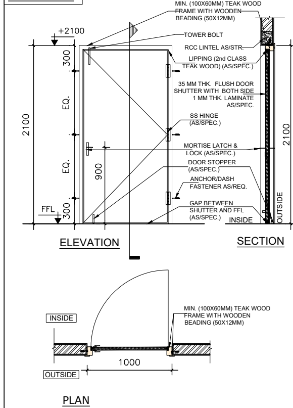
DOOR-D2
