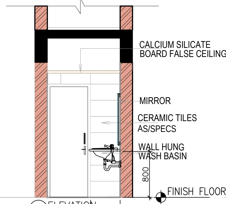
A4 ELEVATION
