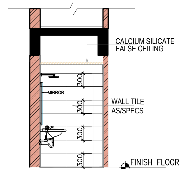
E2 ELEVATION
