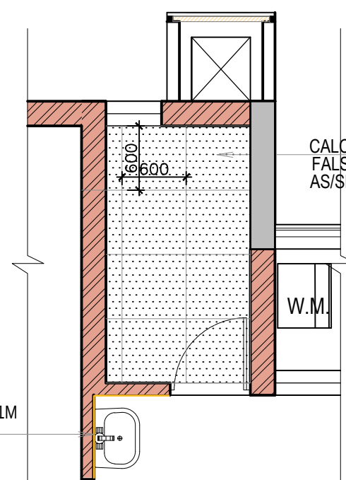
02 PLAN_RCP
