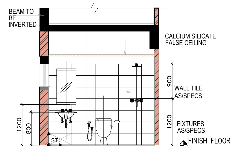
E1 ELEVATION
