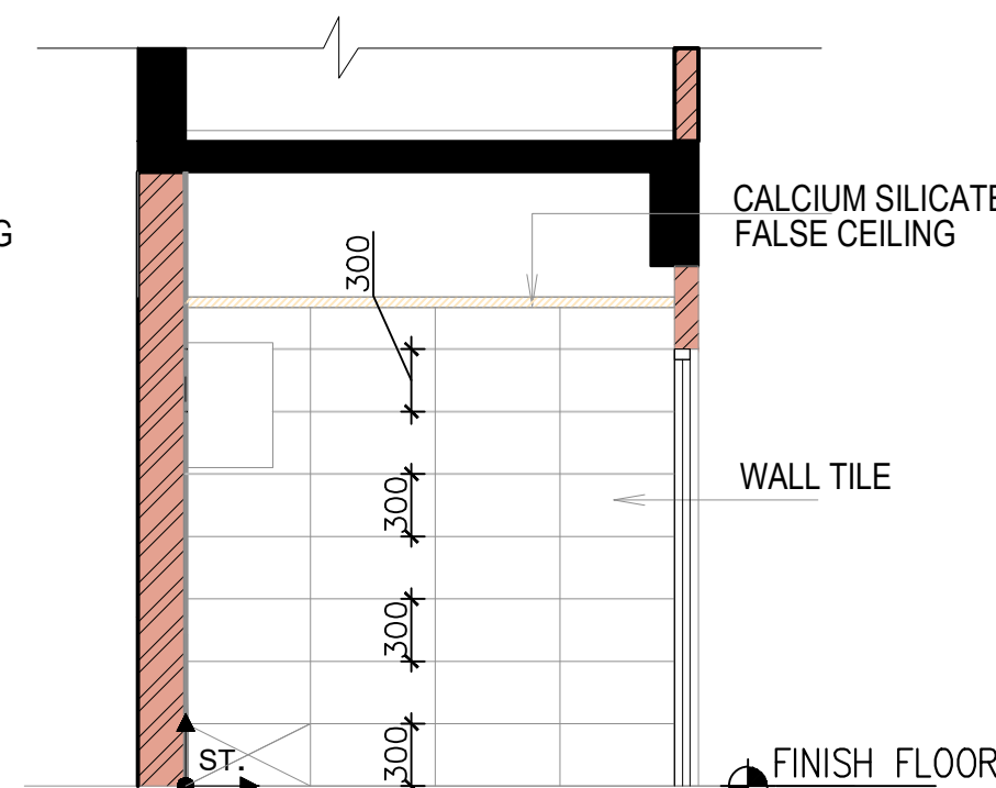
A2 ELEVATION
