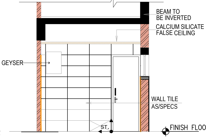
E4 ELEVATION
