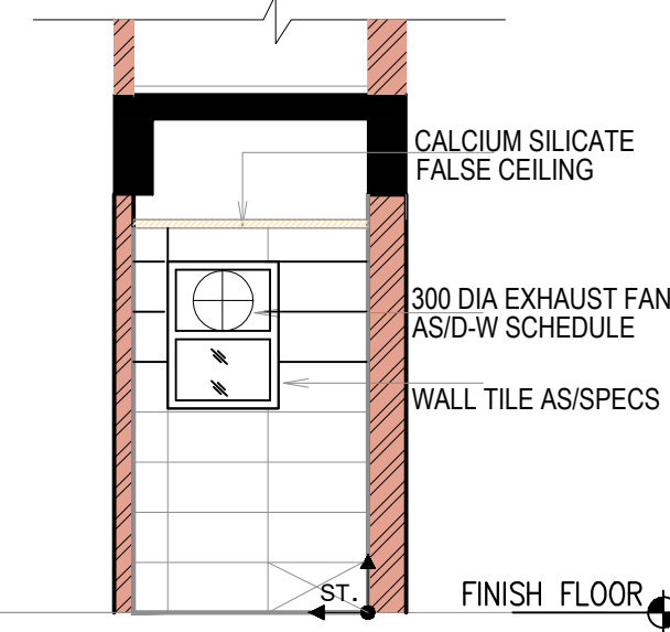
E3 ELEVATION
