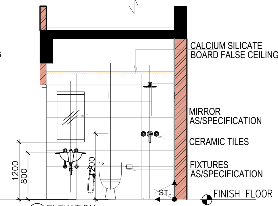
A3 ELEVATION
