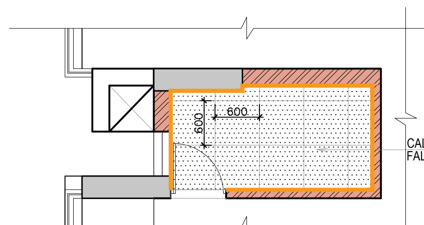
02 PLAN_RCP
