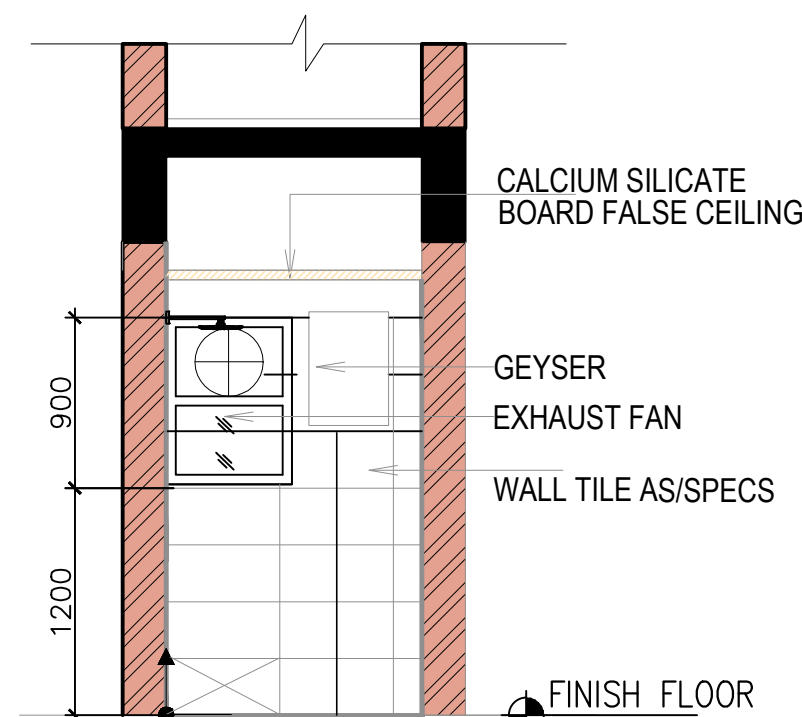
A1 ELEVATION
