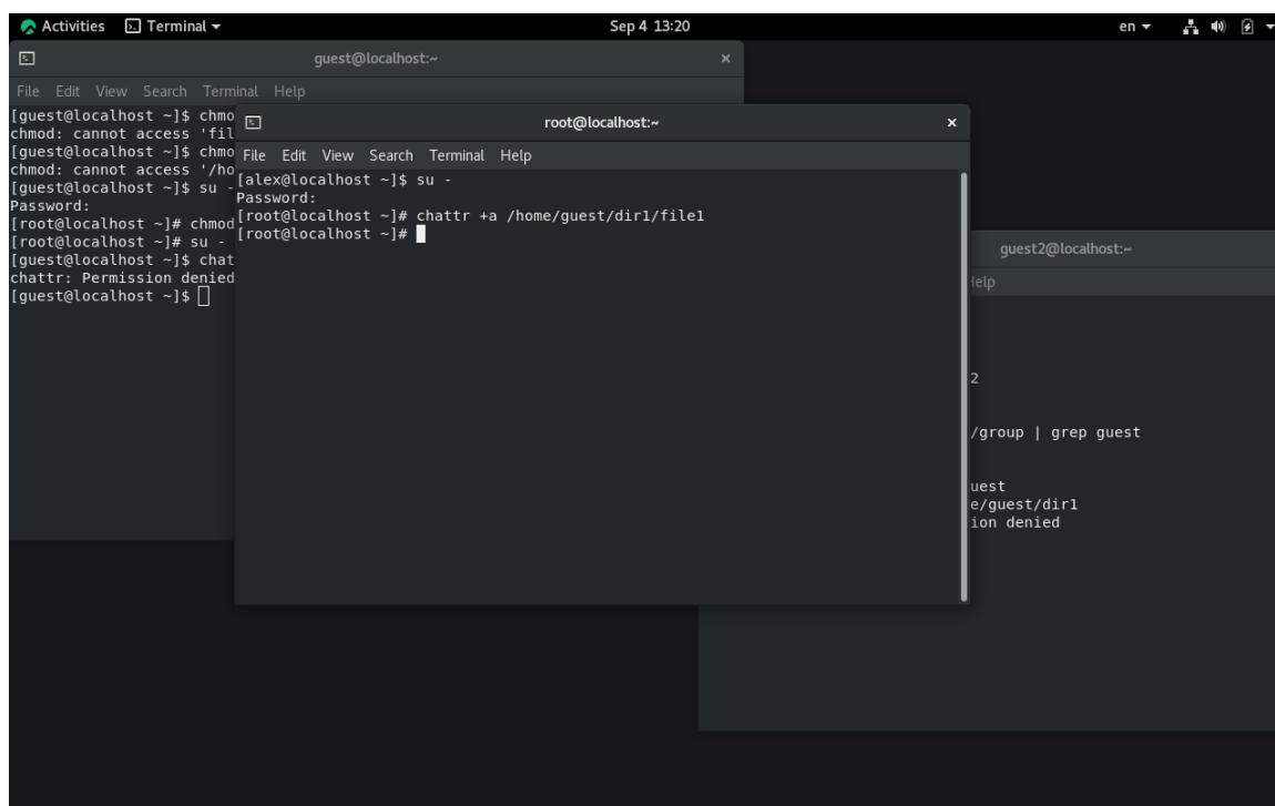
Рисунок 4.4: Установка атрибута а от суперпользователя
