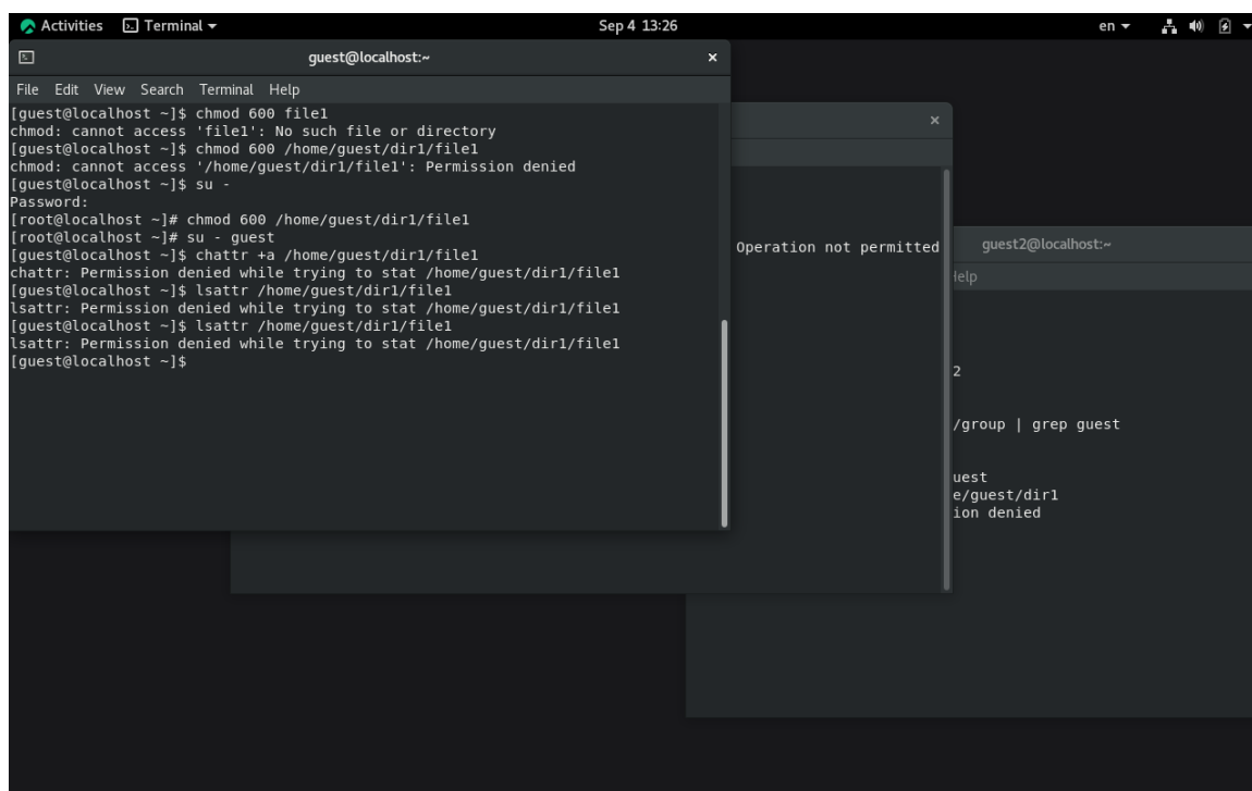
Рисунок 4.5: Проверка установки расширенного атрибута
