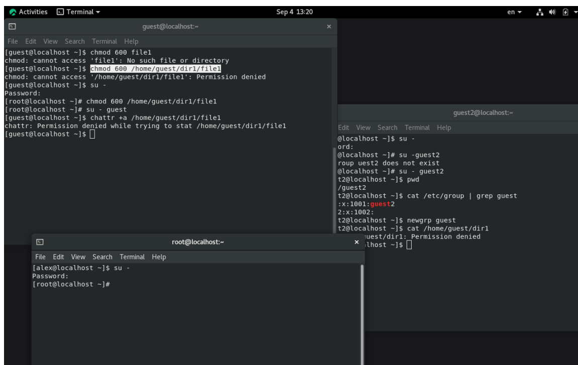
Рисунок 4.3: Попытка установки атрибута от обычного пользователя
