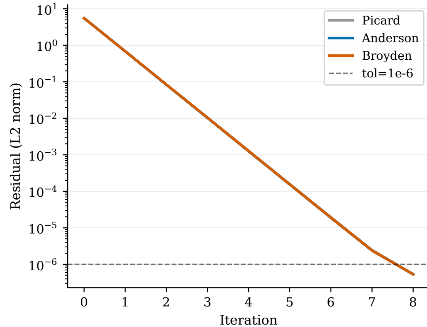
Dimension 512
