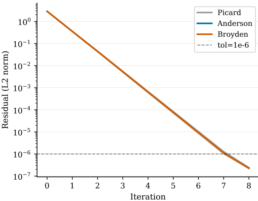
Dimension 128
