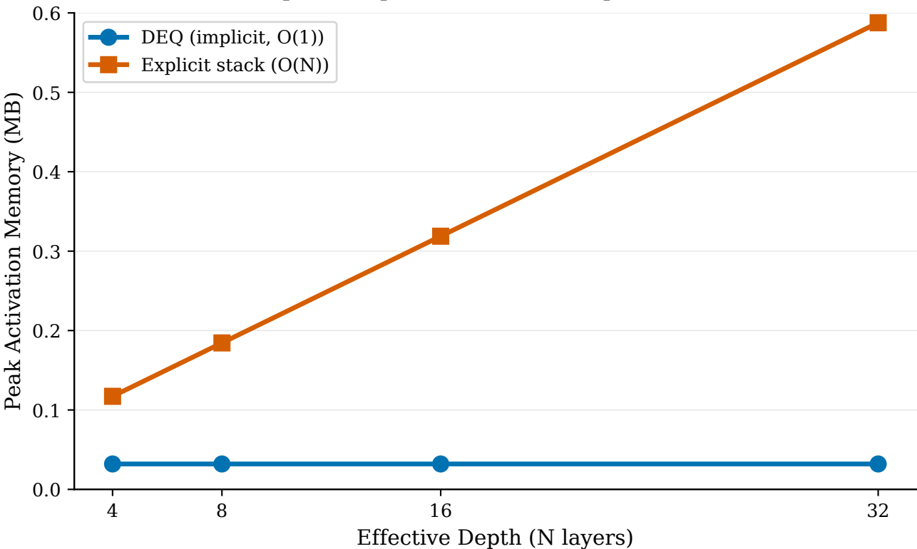
DEQ: Implicit Depth Scales O(1) ; Explicit Scales O(N)
