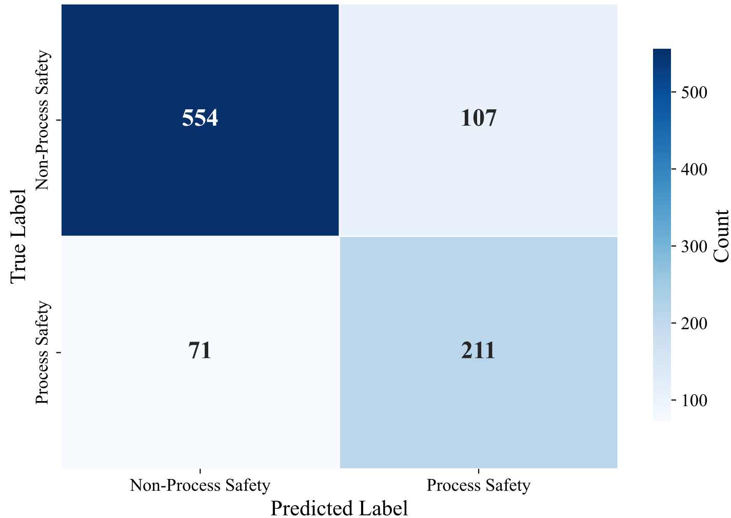
Confusion Matrix — MANUAL (BERT + SVM)
