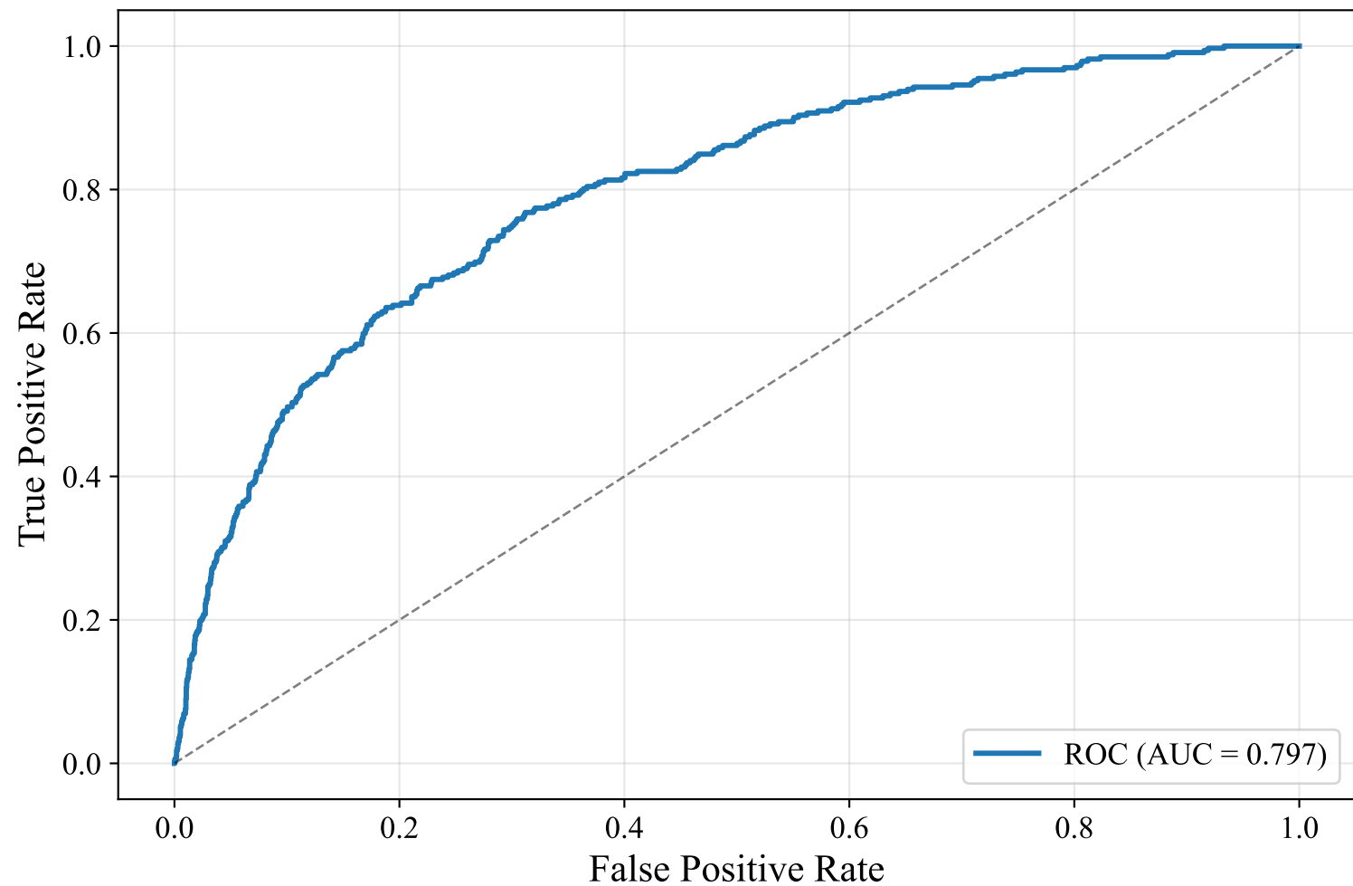
ROC Curve — GERMAN_MANUAL (bert-base-multilingual-uncased, SVM)
