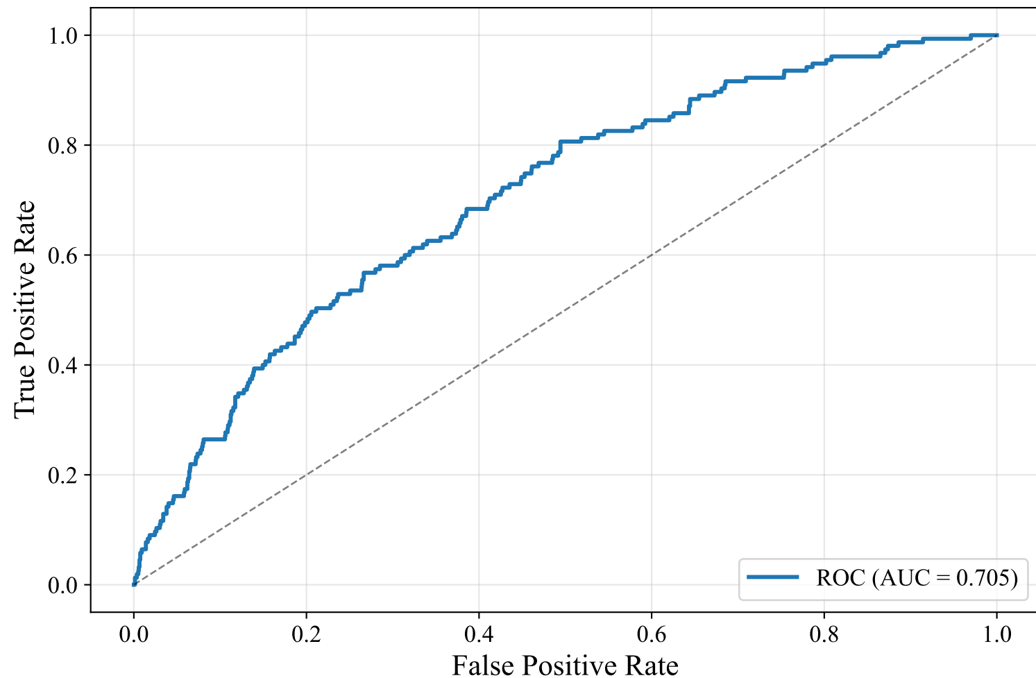
ROC Curve — SWEDEN_MANUAL (bert-base-multilingual-uncased, SVM)
