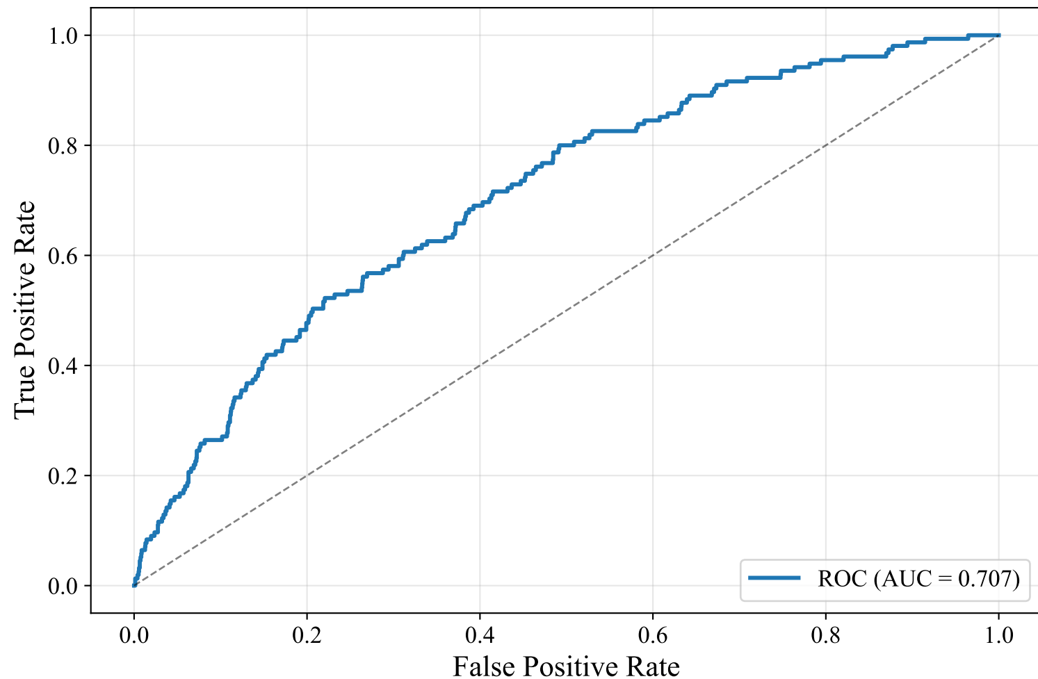
ROC Curve — SWEDISH_MANUAL (bert-base-multilingual-uncased, SVM)
