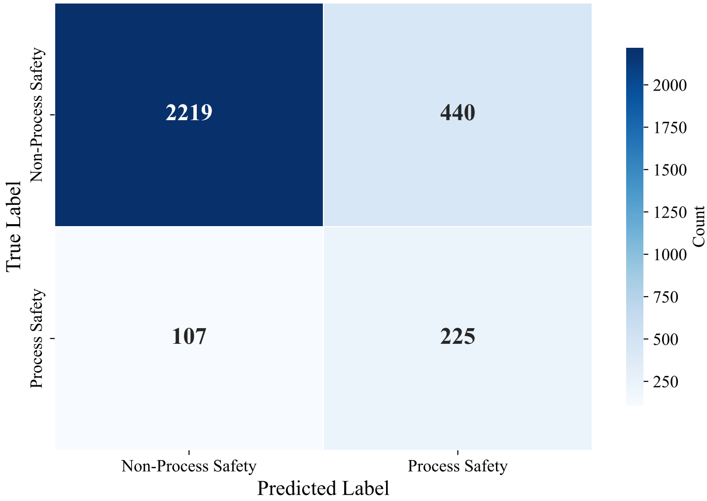
Confusion Matrix — GERMAN_MANUAL (bert-base-multilingual-uncased, SVM)
