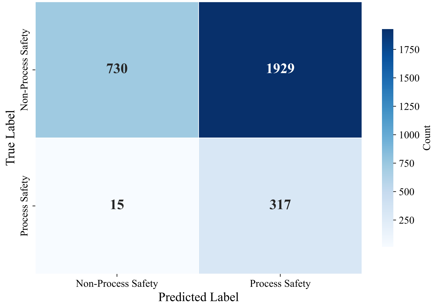
Confusion Matrix — GERMAN_MANUAL (bert-base-multilingual-uncased, svm_rbf)
