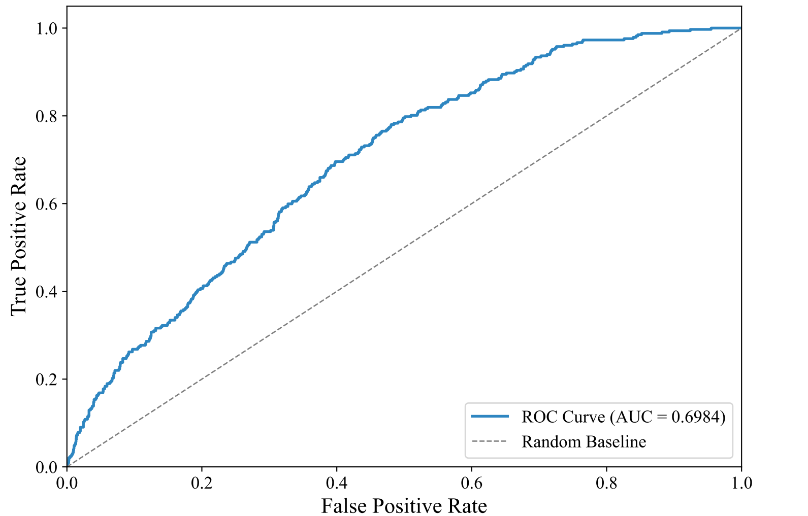
ROC Curve — GERMAN_MANUAL (bert-base-multilingual-uncased, svm_rbf)
