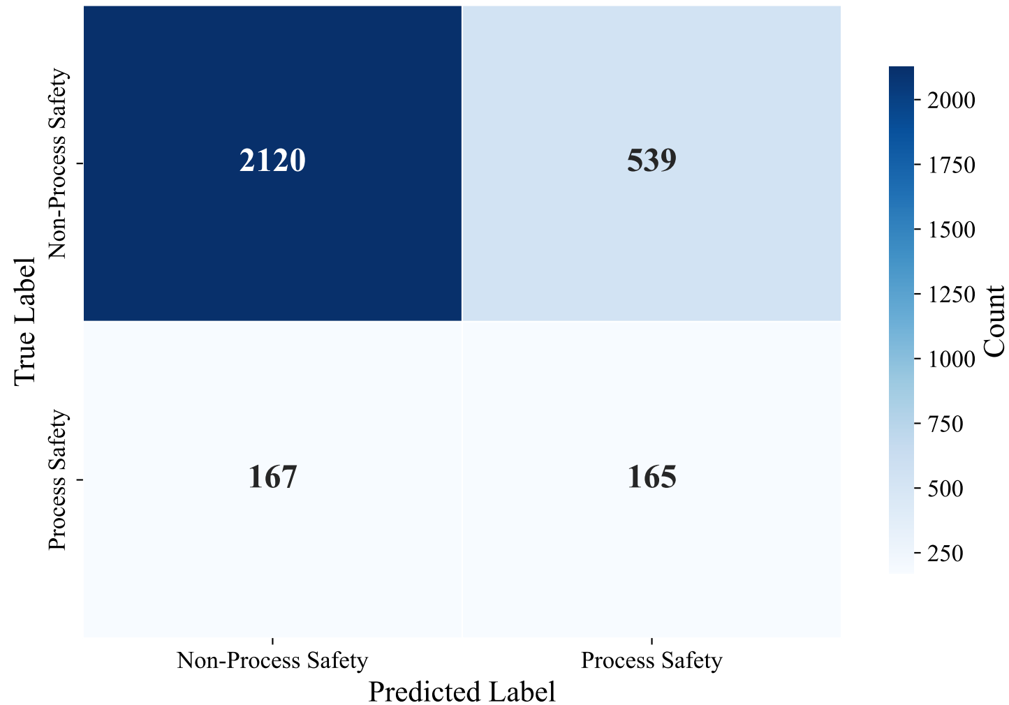
Confusion Matrix — GERMANY_MANUAL (bert-base-cased)
