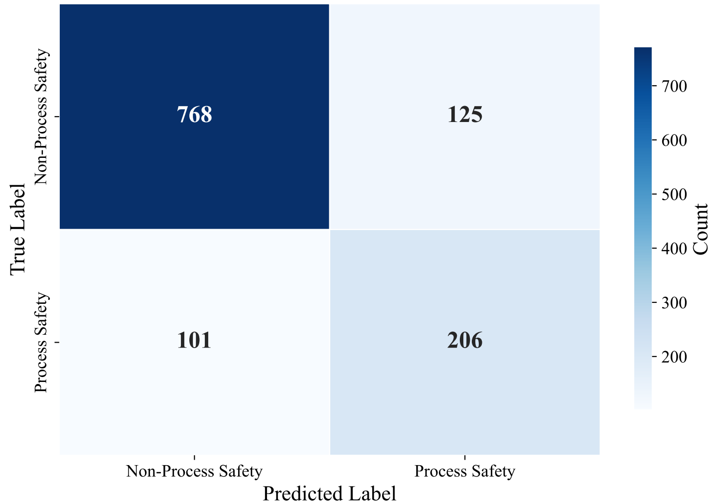
Confusion Matrix — LANGDETECT (BERT + SVM)
