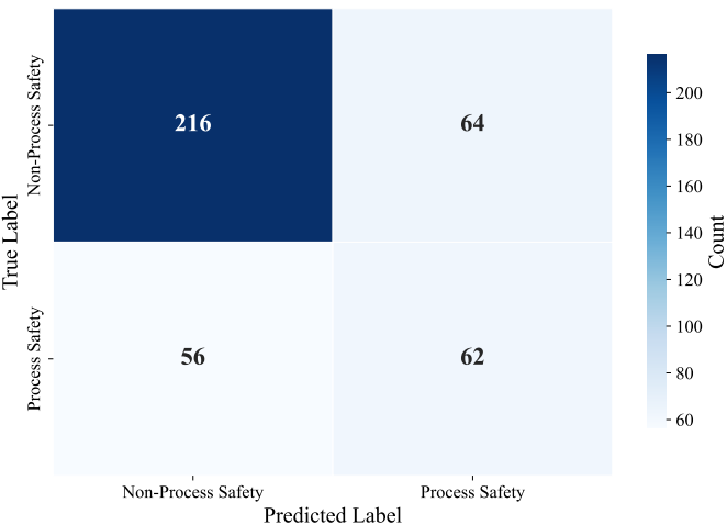
(d) roberta-base.
