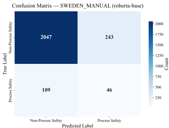
(d) roberta-base.
