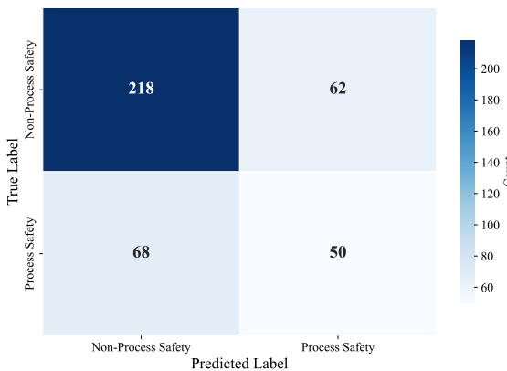
(d) intfloat_multilingual-e5-large.
