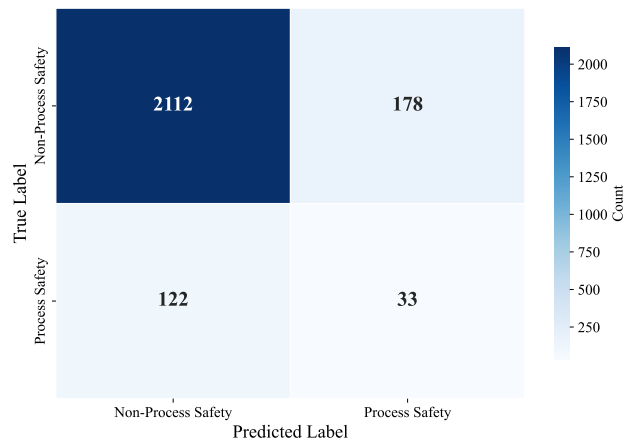
(d) intfloat_multilingual-e5-large.
