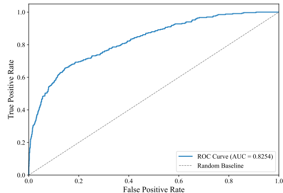
(d) ROC Curve.
