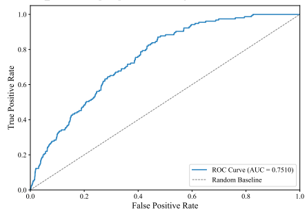
(d) ROC Curve.
