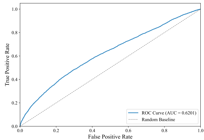
(d) ROC Curve.
