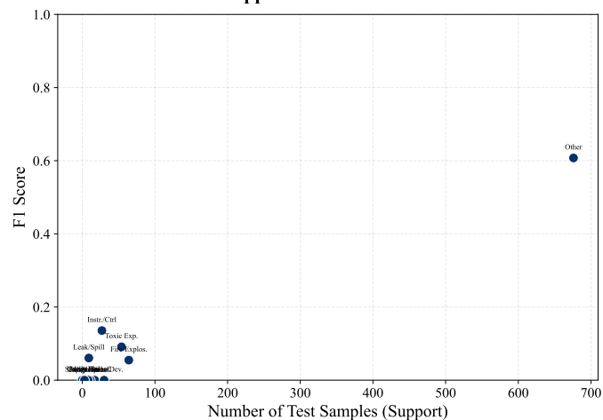
(d) support vs f1.
