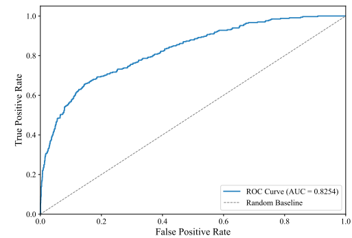
(d) ROC Curve.
