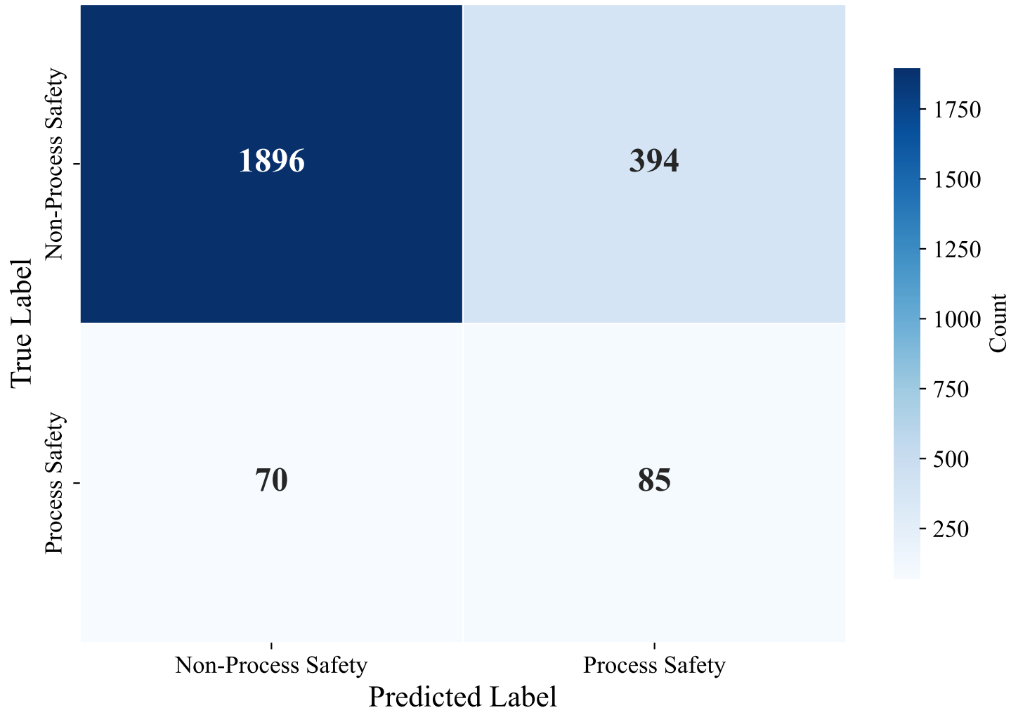
Confusion Matrix — SWEDISH_MANUAL (bert-base-multilingual-uncased, SVM)
