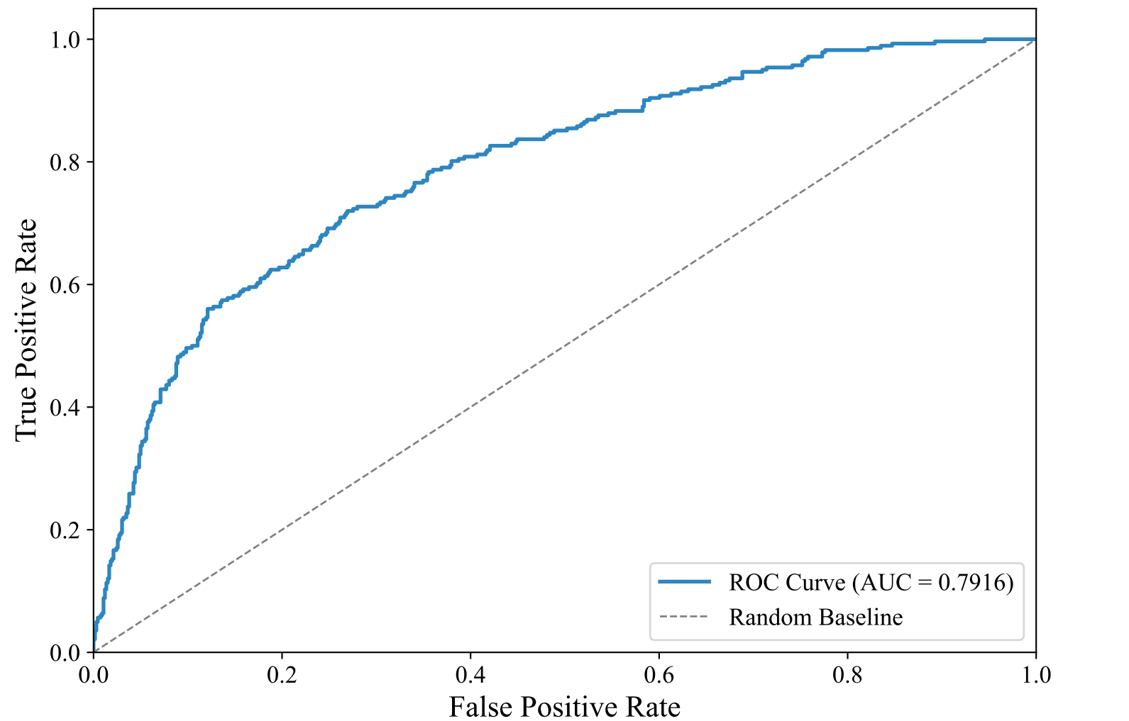
ROC Curve — ENGLISH_MANUAL (bert-base-multilingual-uncased, svm_rbf)
