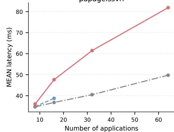
papageissvri
