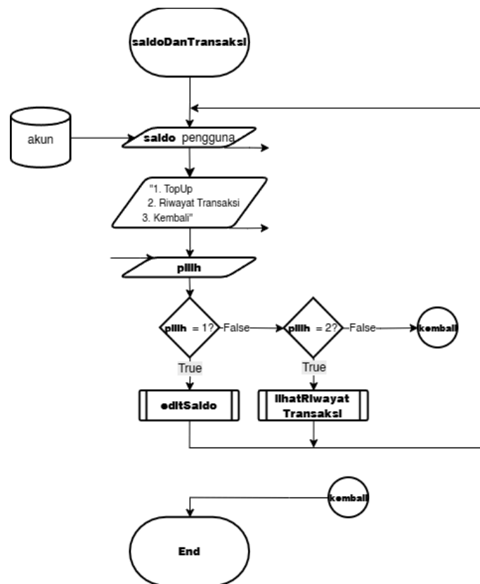
Gambar 2.3.20 Flowchart Menu_saldoDanTransaksi
