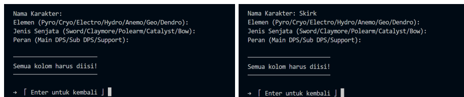
Gambar 4.21. Input Kosong
