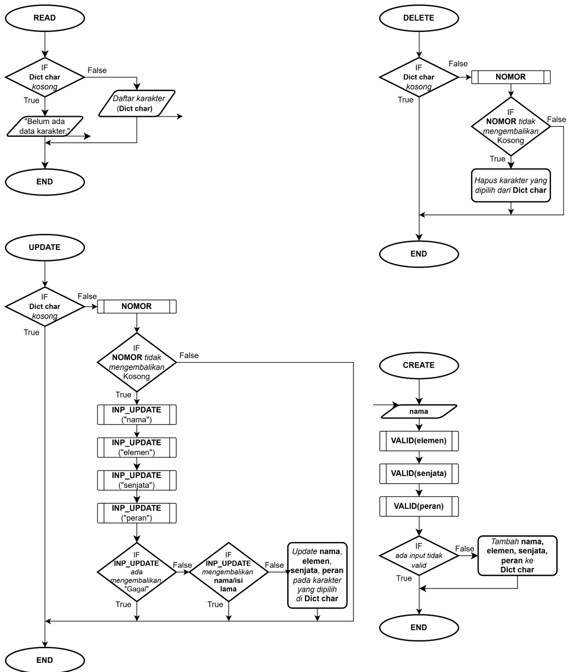
Diagram 1.3. Flowchart Fungsi pada File CRUD Halaman 1
