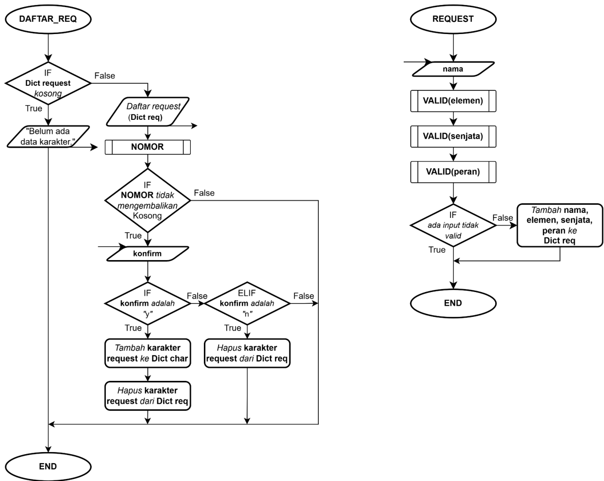
Diagram 1.4. Flowchart Fungsi pada File CRUD Halaman 2
