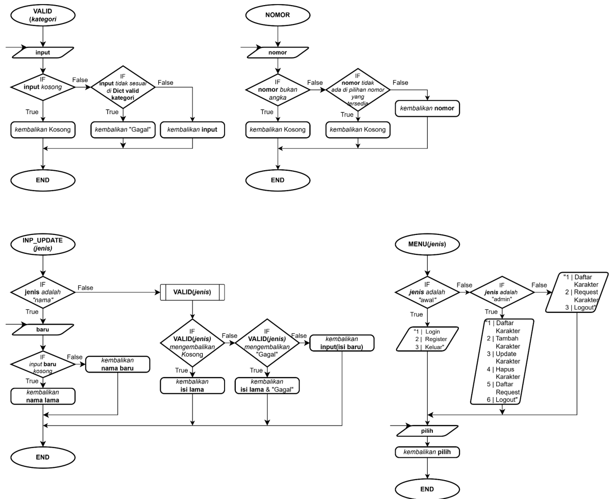
Diagram 1.1. Flowchart Fungsi pada File Menu
