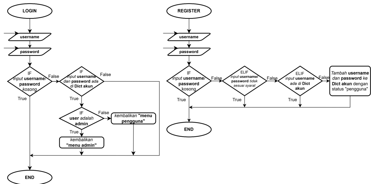
Diagram 1.2. Flowchart Fungsi pada File Autent
