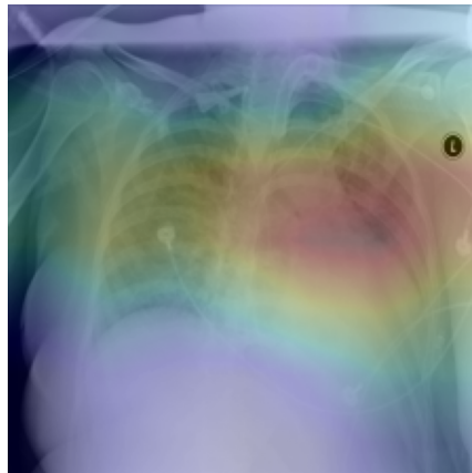
Grad-CAM++ CTI=0.541
