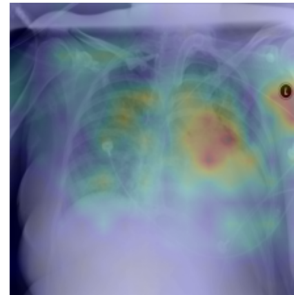
Layer-CAM CTI=0.518
