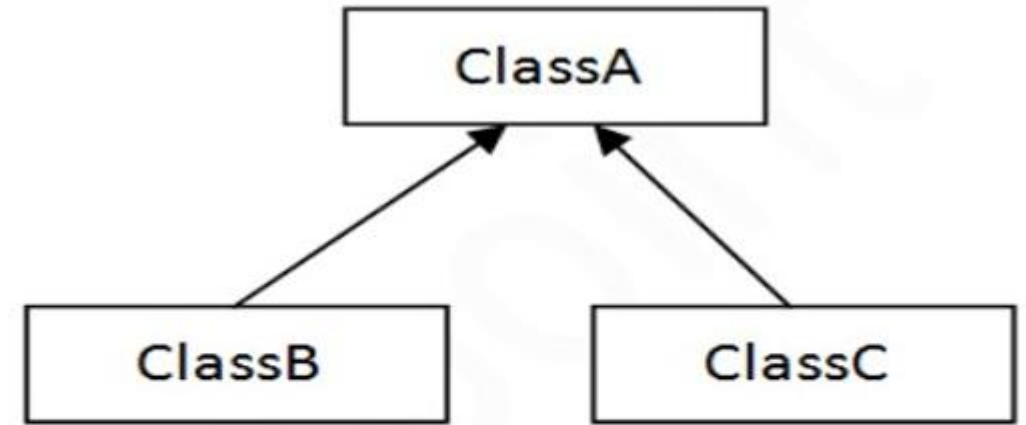
3) Hierarchical
