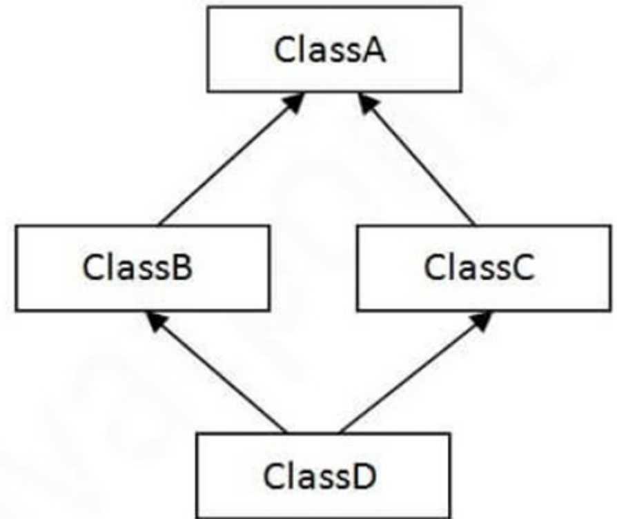
5) Hybrid
