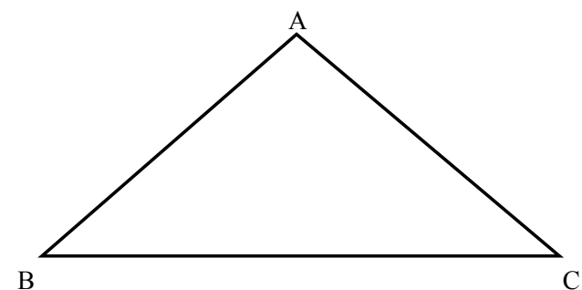
Рис. 1. Треугольник ABC.
