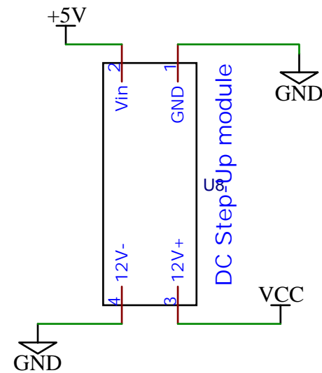
Mini Voltage Converter Step-Up Module 5V 8V 9V 12V Power Boost Convert Module
