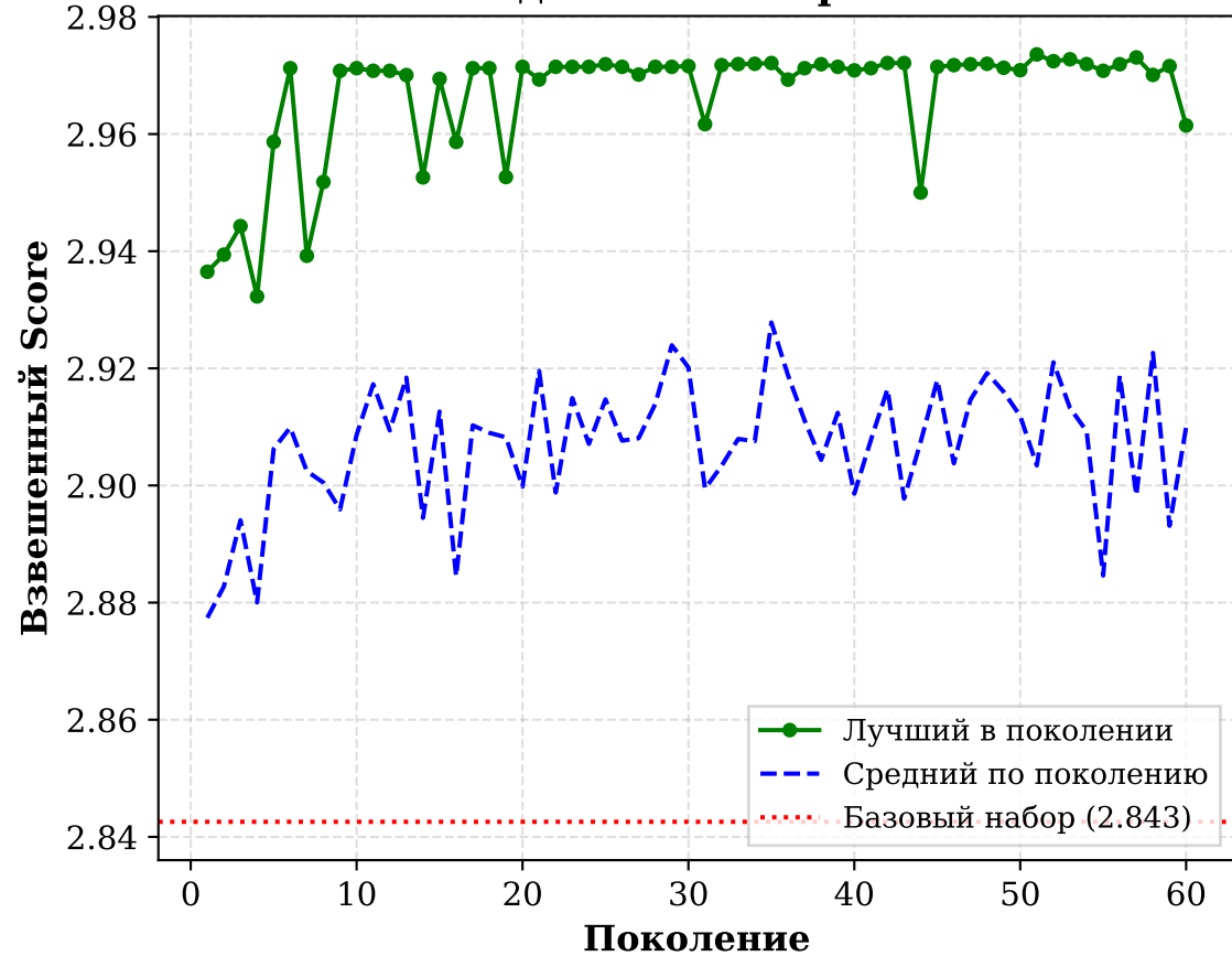
Сходимость алгоритма
