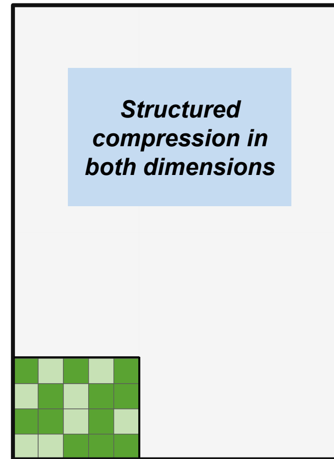
DecoMoE (Ours)
