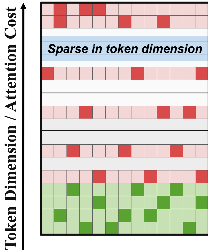
Token Pruning
