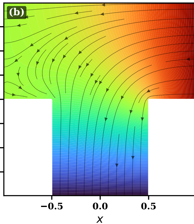
INI-VPINN
