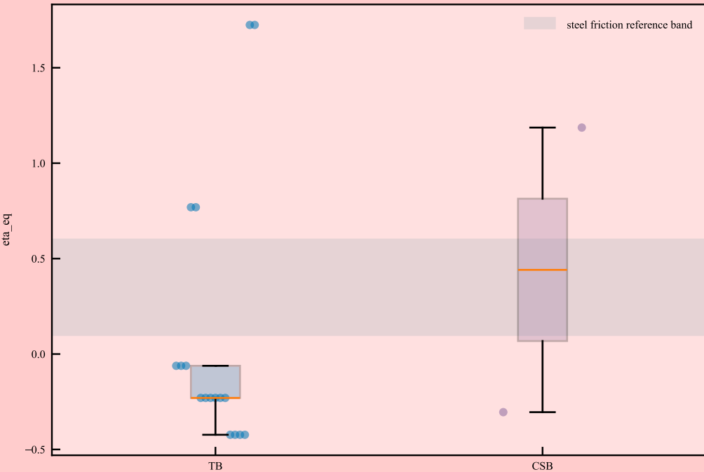
Equivalent Dissipation Parameter Inversion (eta_eq)
