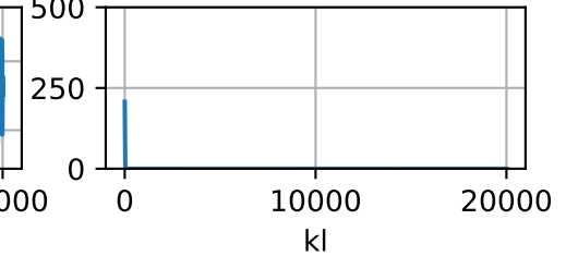
sigma_y=10.0
