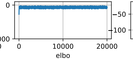
sigma_y=10.0
