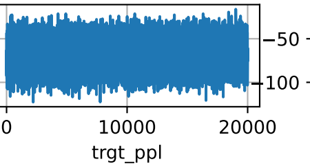
sigma_y=10.0
