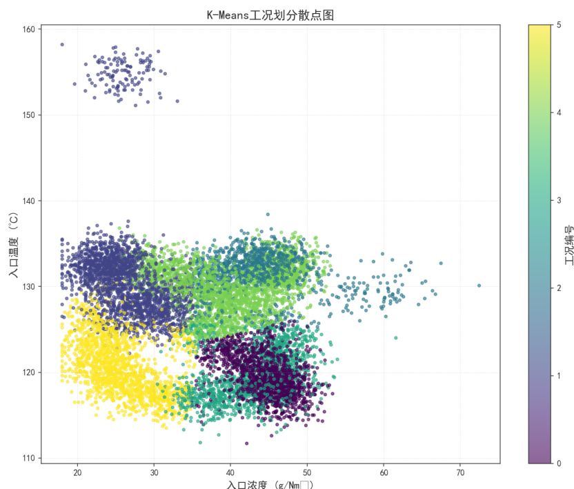
图 2 K-Means 工况划分散点图
