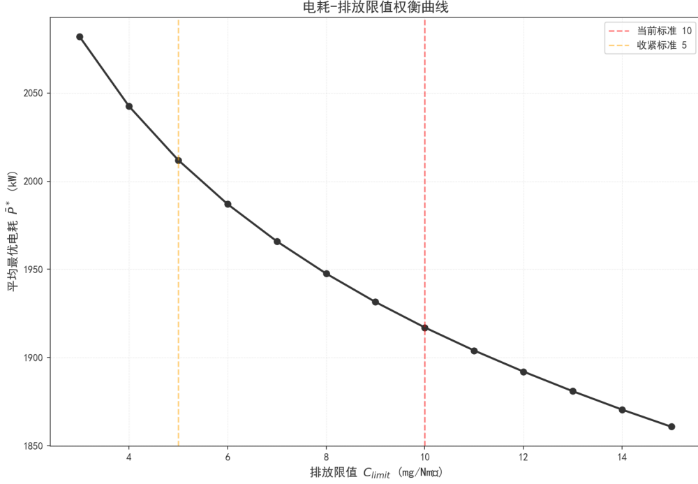
图 6 排放限值连续扫描的电耗-约束权衡曲线
