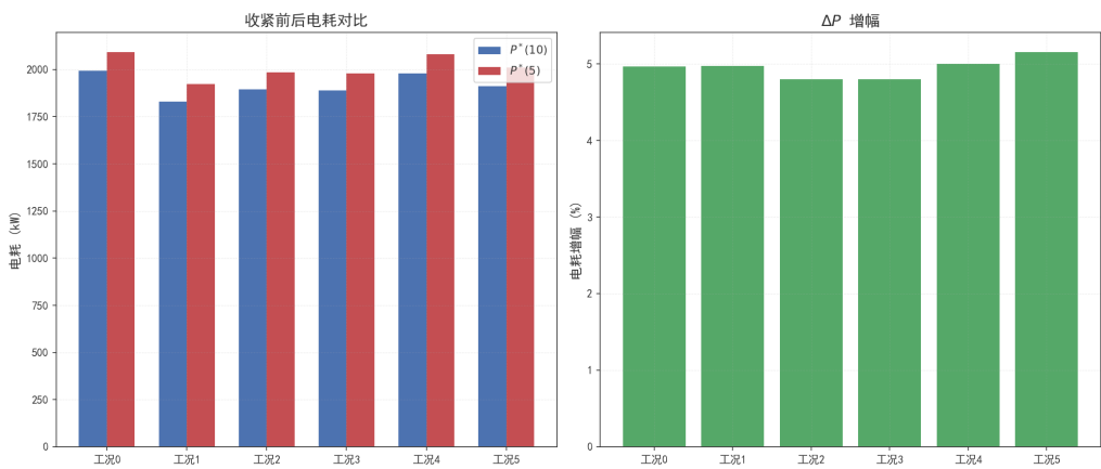
图 5 排放收紧前后各工况电耗对比与增幅
