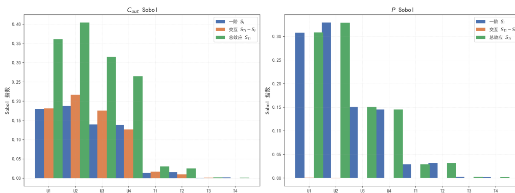
图 7 Sobol 全局灵敏度分析
