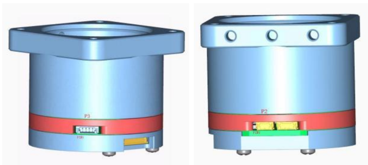
图 2-4 整机接口 2
