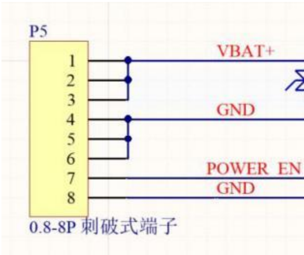
图 2-5 电源接口
