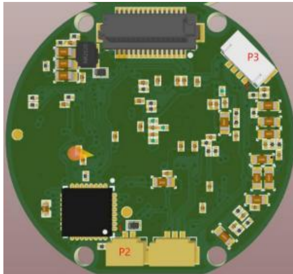
图 2-2 PCB 背面
