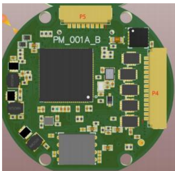
图 2- 1 PCB 正面
