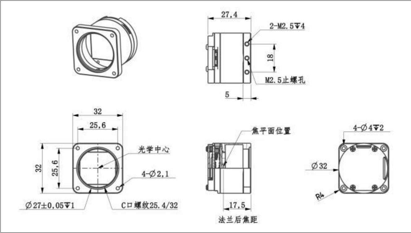
图 2-9 整机结构尺寸
