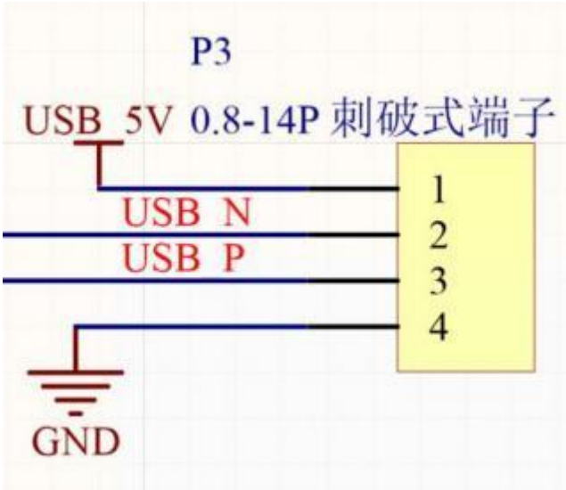
图 2- 8 USB 接口定义
