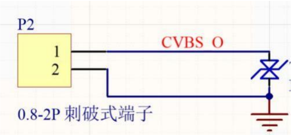
图 2- 7 CVBS 信号
