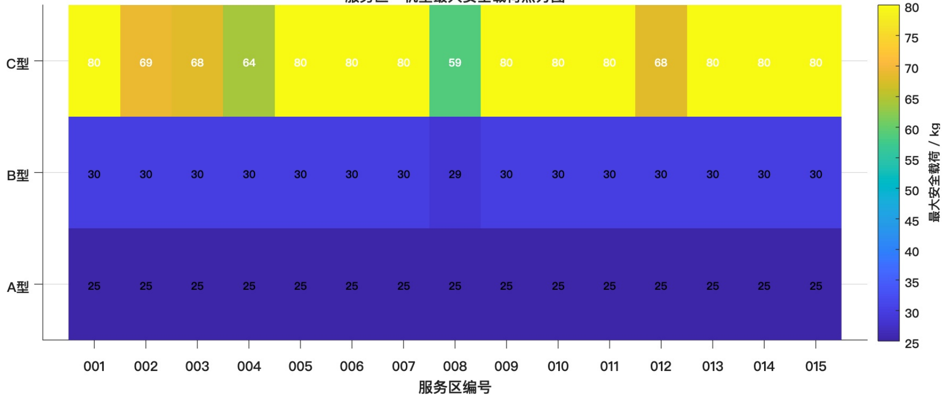
服务区一机型最大安全载荷热力图
