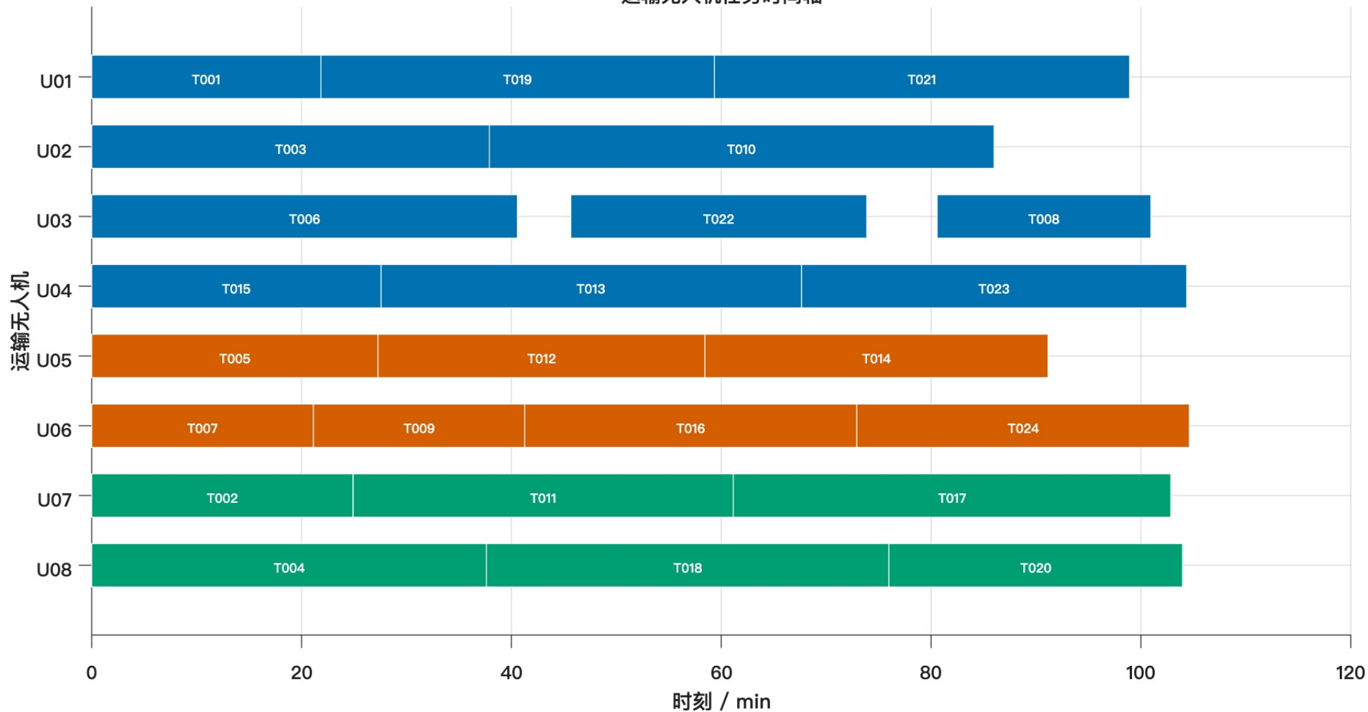
运输无人机任务时间轴
