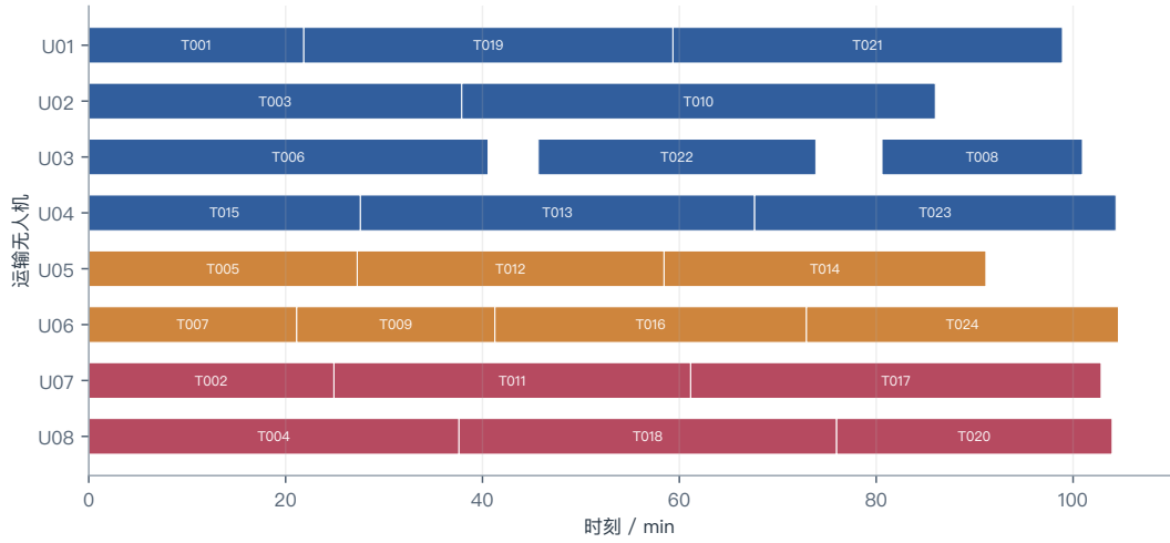
图 5: 问题二运输机架次时间表
