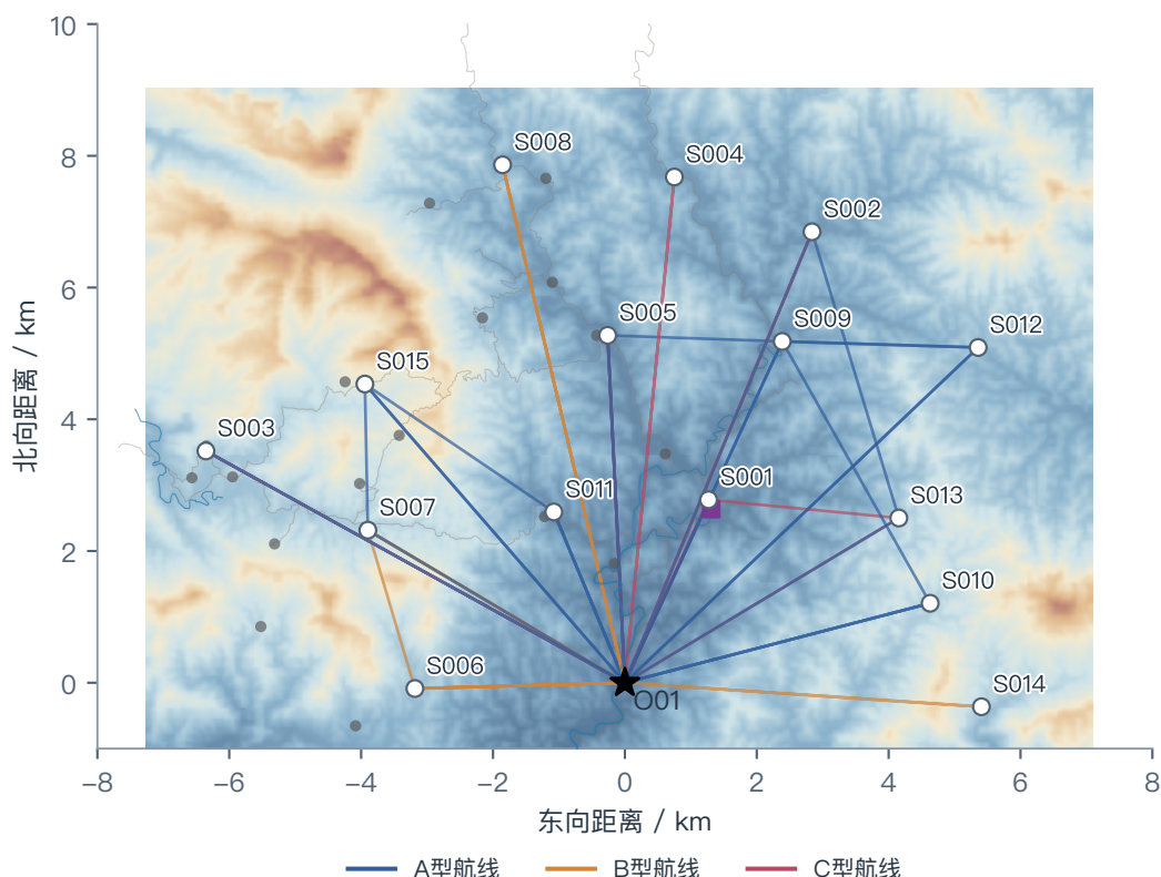
图 4: 问题二多点运输航线与服务区位置
