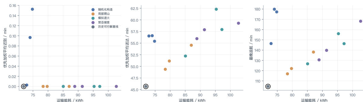
图 3: 修订时限后的同预算算法：耗电与加权迟到、交付和最后返航；黑圈为提交方案
