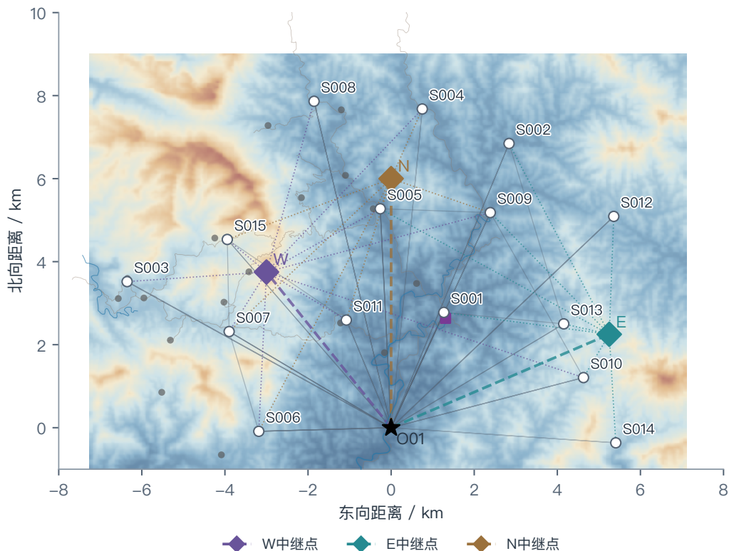
图 6: 主方案西、东、北中继悬停点
